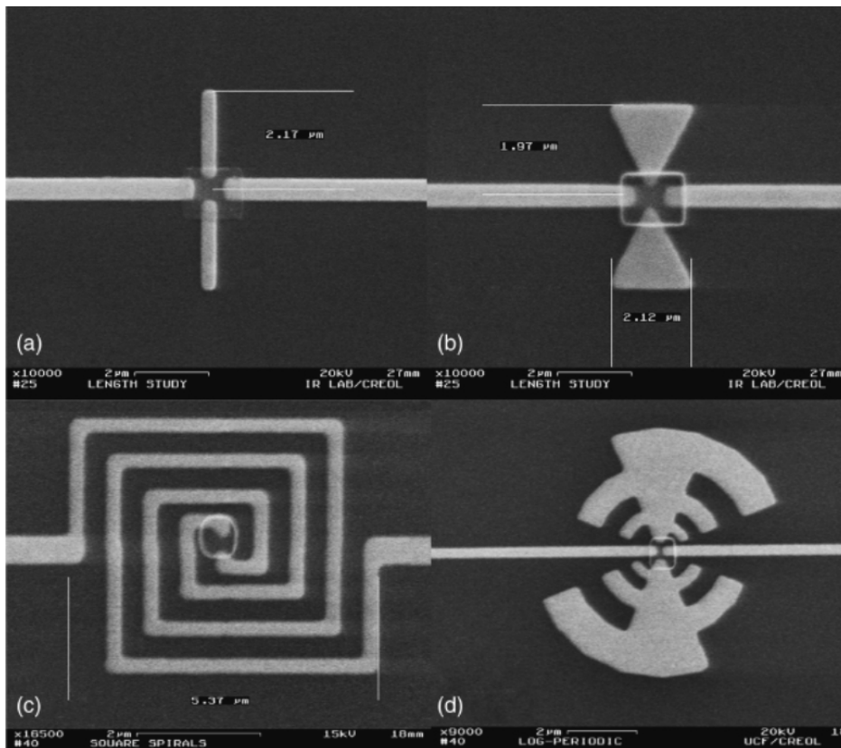
Figura1: Nanoantenas fabricadas usando litografía por haz de electrones. Se muestran diferentes geometrías: (a) dipolo, (b) corbata, (c) espiral, (d) antena log-periódica [3].
